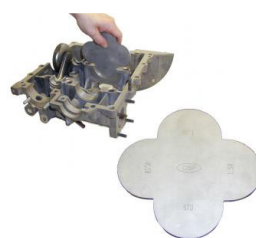
Carter hoofdlager 1-3 meet hulpstuk type-1 motor (behalve 25pk en 30pk), type-3 motor, CT/CZ motor, Waterboxer motor
