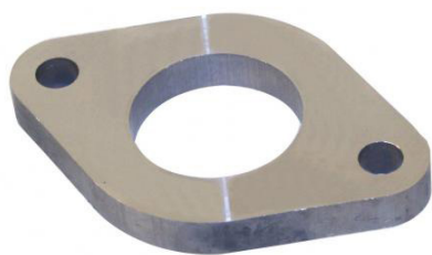
Carburateur verhogings adapter (9 mm) Voor standaard 34 PICT carburateurs
