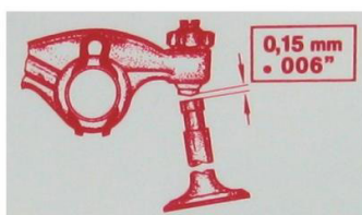
Sticker klepspeling Kever 8.1964 en later, Karmann Ghia 8.1964 en later, Bus 8.1967 t/m 7.1973 met 1700cc motor, type-3 8.1964 en later, Kübel
